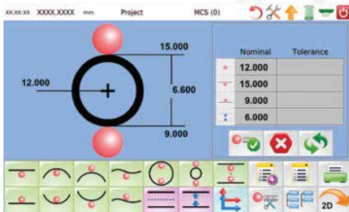
▲ Esempi di misurazione. Example: measurement.
